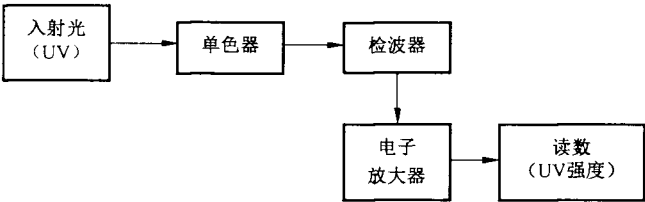
图 3 测试原理图
